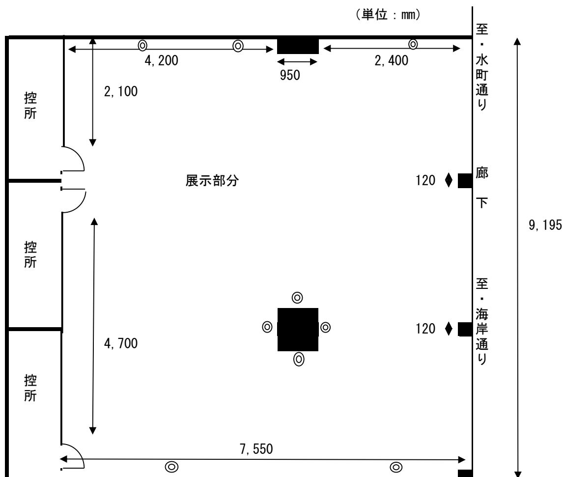
ギャラリースペース平面図
